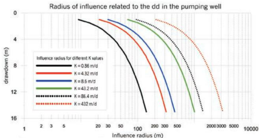
Slika 4-3 Varijacija radijusa utjecaja uslijed promjene hidrauličke vodljivosti i pada razine podzemne vode (Fileccia, 2015)
