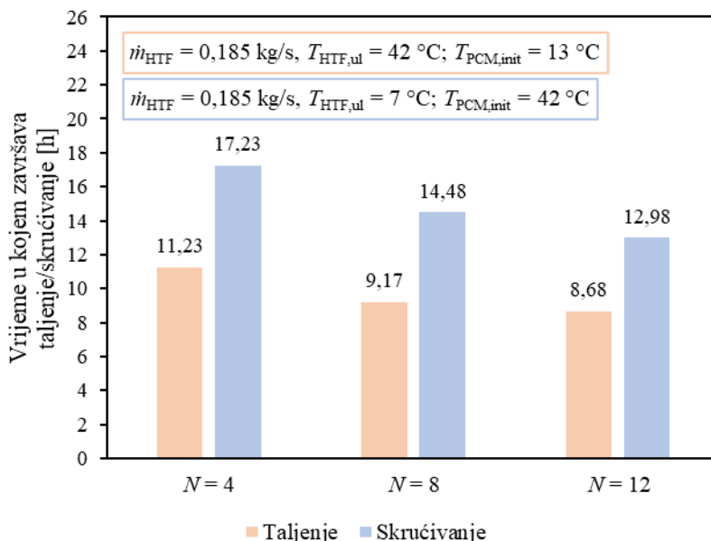
Slika 8.7. Usporedbe vremena u kojima završavaju taljenje/skrućivanje dobivenih numeričkim proračunima za analizirane brojeve lamela
