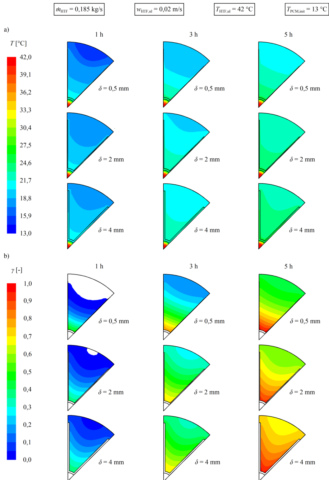
Slika 8.15. Usporedba raspodjela temperatura (a) i udjela kapljevite faze (b) u ravnini xy za z = 0,75 \text{ m} prilikom spremanja topline dobivenih numeričkim proračunima u proračunskim vremenima 1, 3 i 5 h za konfiguracije latentnog spremnika topline s lamelama debljine 0,5, 2 i 4 mm
