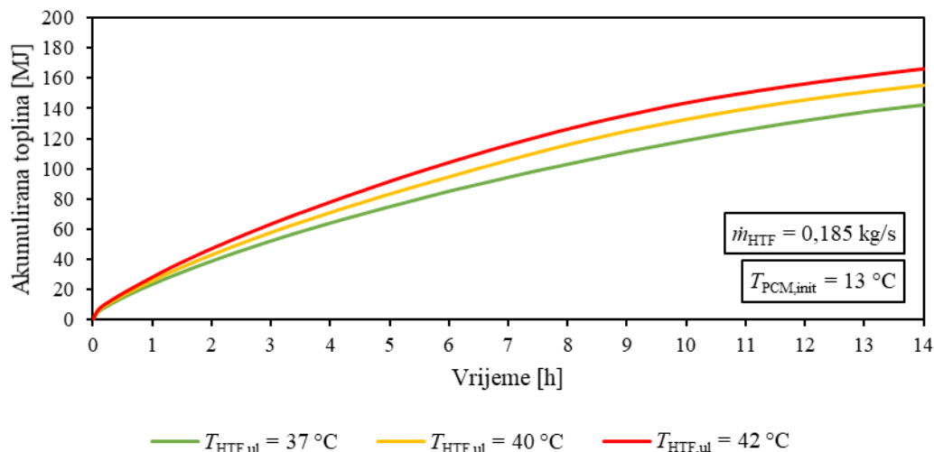
Slika 4.4. Vremenske promjene akumuliranih toplina prilikom spremanja topline dobivene rezultatima eksperimentalnih mjerenja za različite ulazne temperature fluida prijenosnika topline
