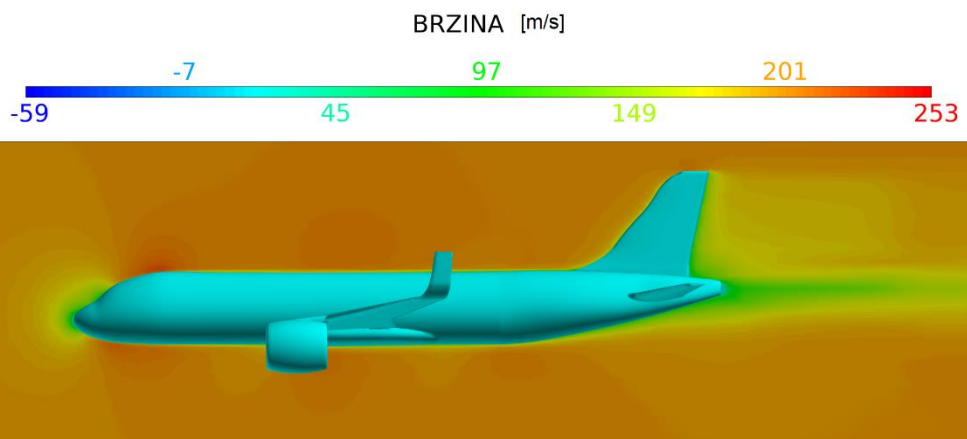
Slika 3.40 Brzine - Bočni pogled - 200 m/s i 0^\circ
