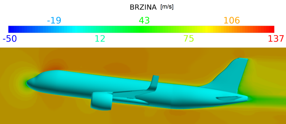
Slika 3.41 Brzine - Bočni pogled - 100 m/s i 7^\circ
