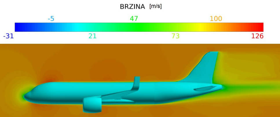
Slika 3.39 Brzine - Bočni pogled - 100 m/s i 0^\circ
