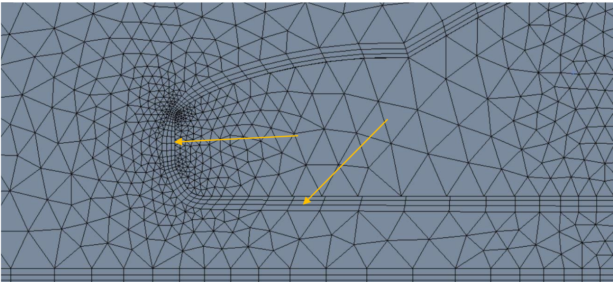
Slika 5.10. Granični slojevi
