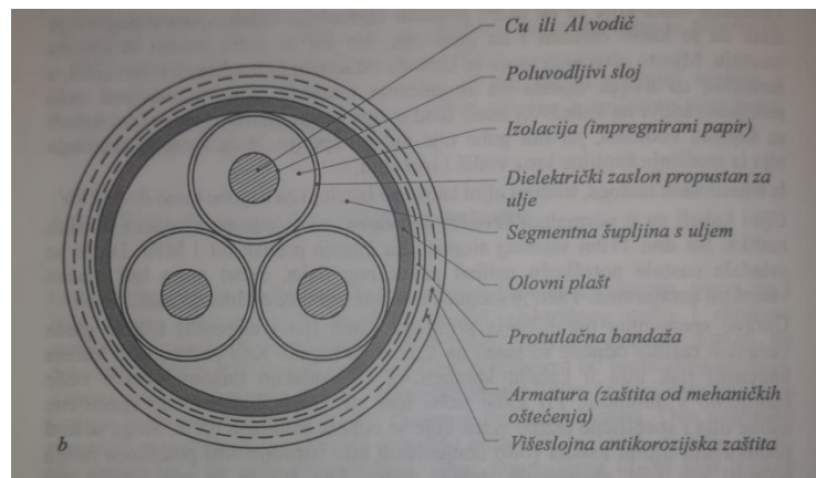
Slika 2.16. Niskotlačni trožilni uljni kabel s armaturom [1]
