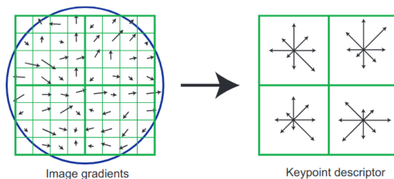
Slika 5: SIFT: gradijenti
