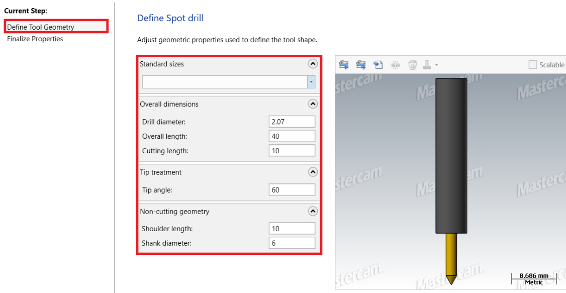
Slika 6.176 dimenzije i izgled kreiranog zabušivača
