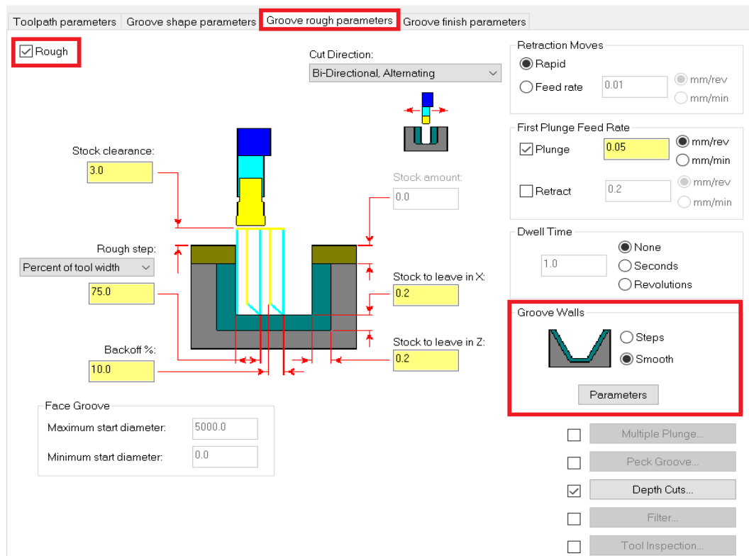
Slika 6.87 Parametri obrade za četrnaesti zahvat
