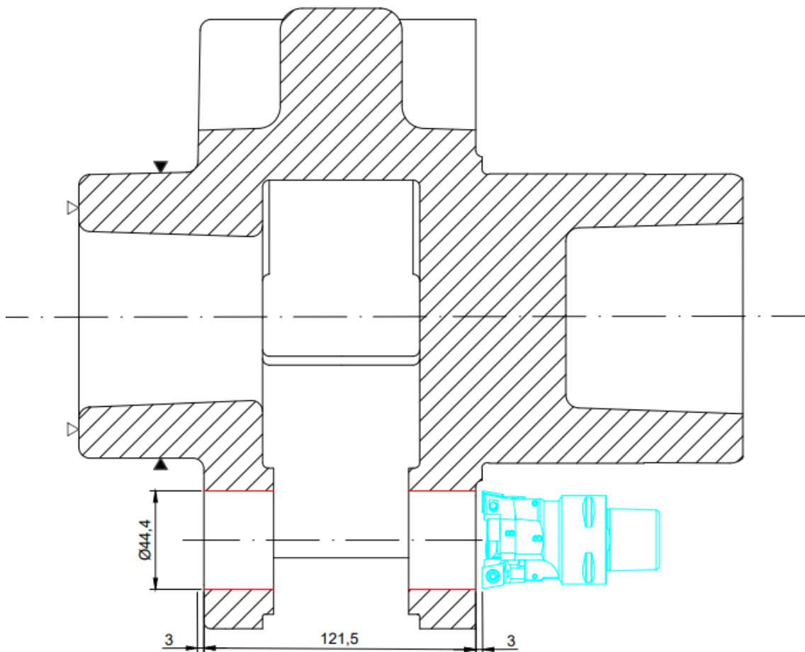
Slika 5.12 Operacija 10 - zahvat 9
