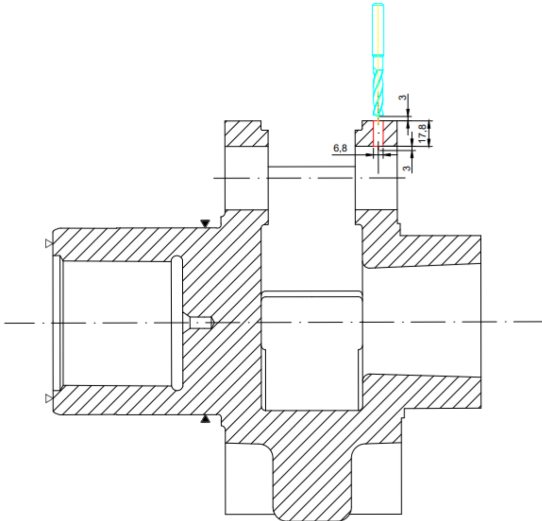
Slika 5.25 Operacija 20 - zahvat 6
