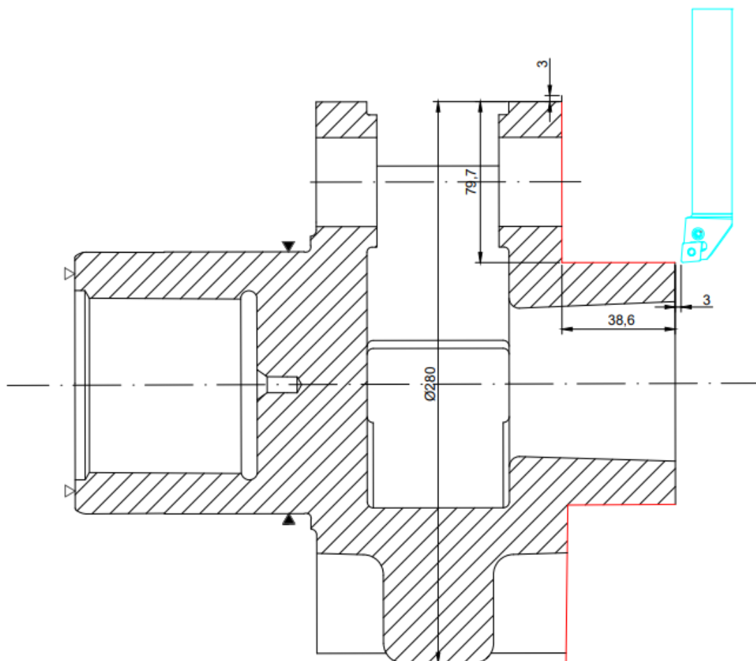
Slika 5.22 Operacija 20 - zahvat 3
