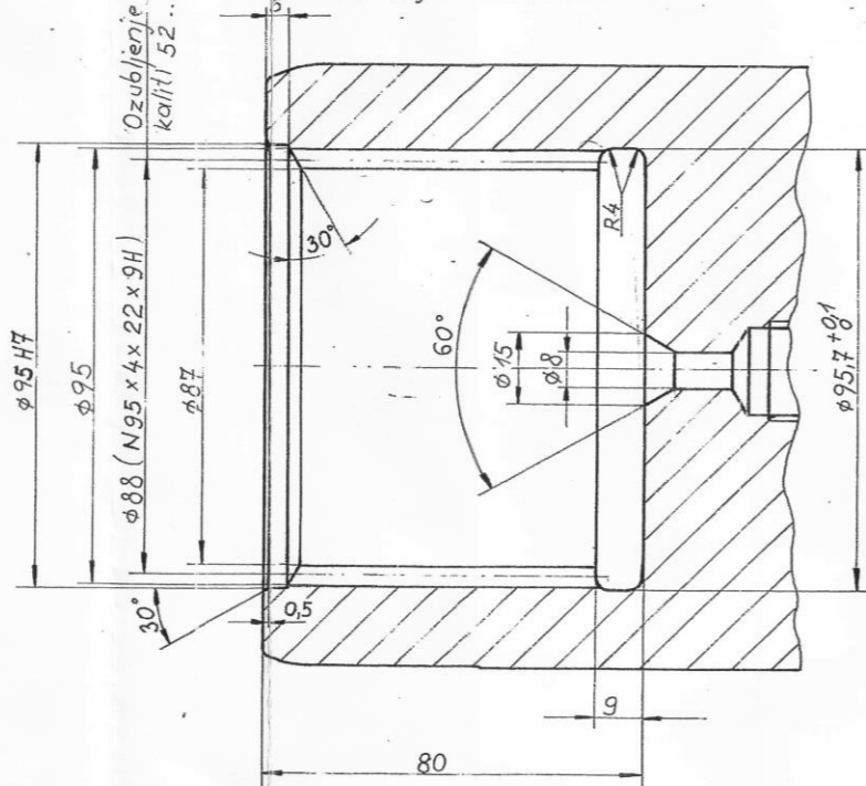
Presjek C-C
