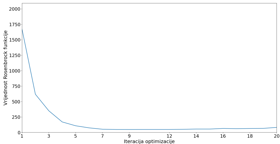
Slika 4.5 Tijek optimizacije (Rosenbrock funkcija s 10 parametara)
