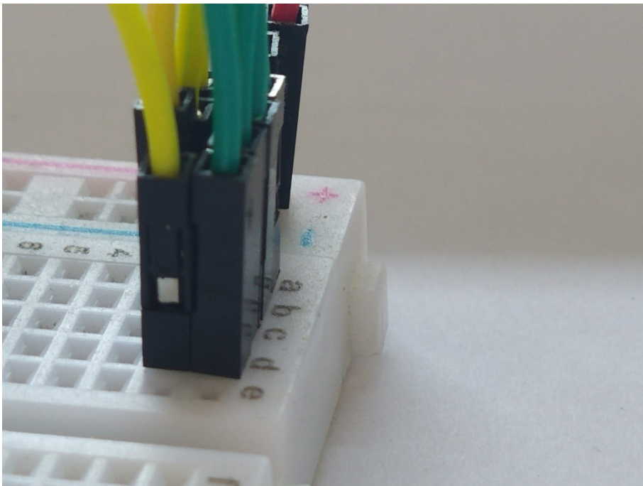
Slika 4.2. Izgled eksperimentalne pločice nakon spajanja \text{FPC} vodiča i vodiča napajanja
