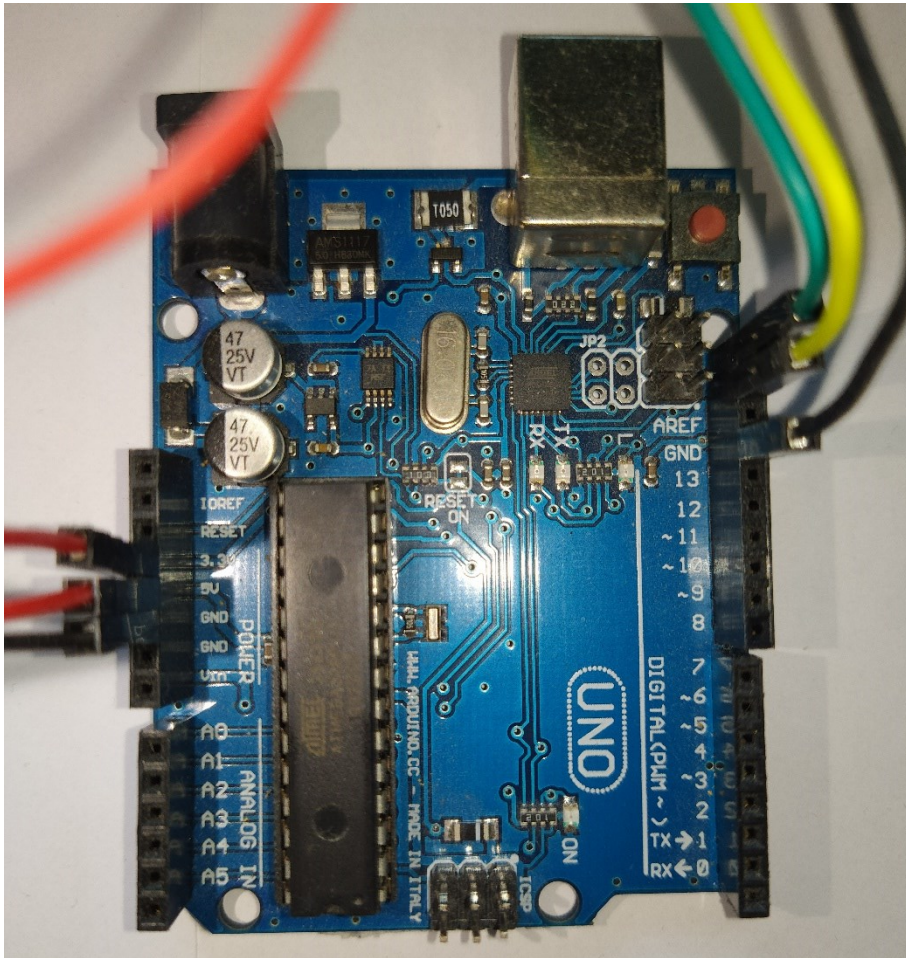
Slika 4.1. Izgled Arduino Uno R3 pločice nakon spajanja vodiča na \text{FPC} ulaze te na ulaze za napajanje i masu
