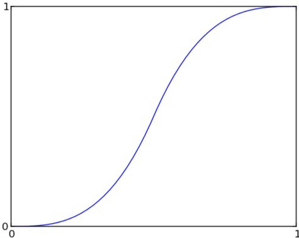
Slika 6.6. Krivulja EaseInOut .
