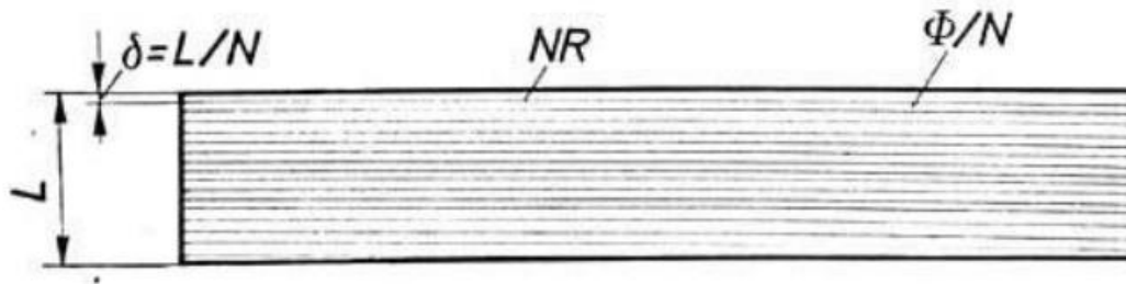
Slika 4.3. Prikaz jezgre transformatora podijeljene na N jednakih dijelova
