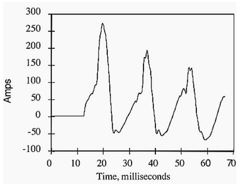
Slika 6.4. - Primjer ulazne struje izmjerene u podstaniци (mnogi distribucijski transformatori zajedno)
