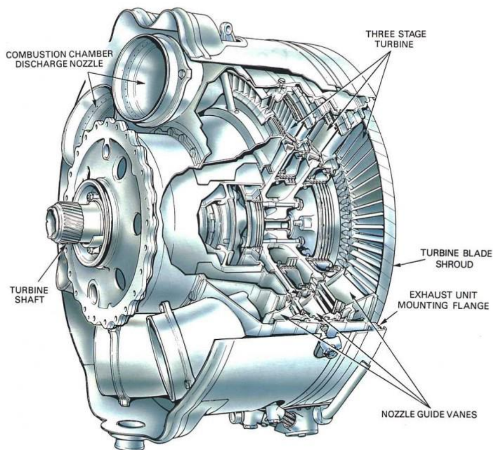
Slika 2.4 Plinska turbina
