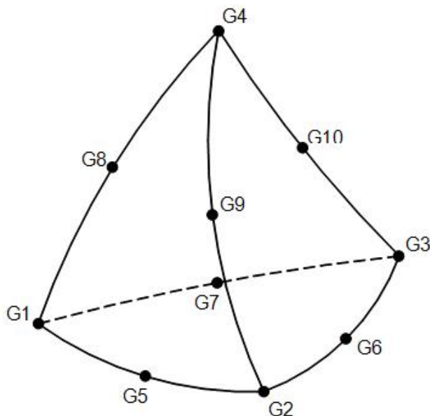
Slika 12. Parabolični tetraedar[9]
