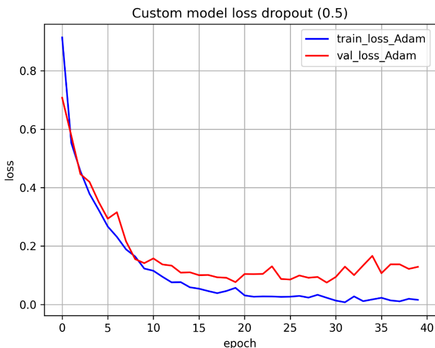
Slika 25. Gubitak prilagođenog modela koristeći dropout(0.5) kod Adam optimizacijskog algoritma
