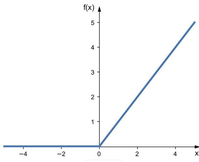
Slika 8. ReLU funkcija [21]
