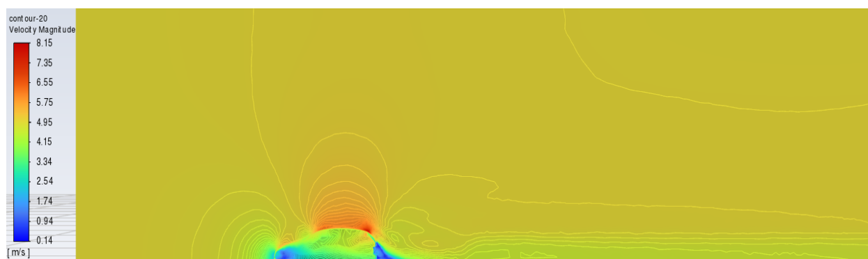
Slika 0.1 Kontura brzina za ulaznu brzinu v = 5 m/s
