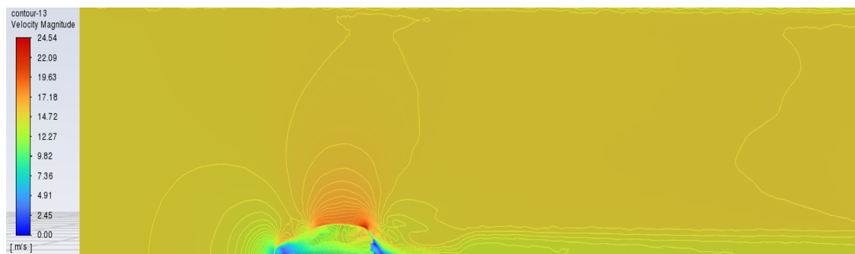
Slika 0.2 Kontura brzina za ulaznu brzinu v = 15 m/s
