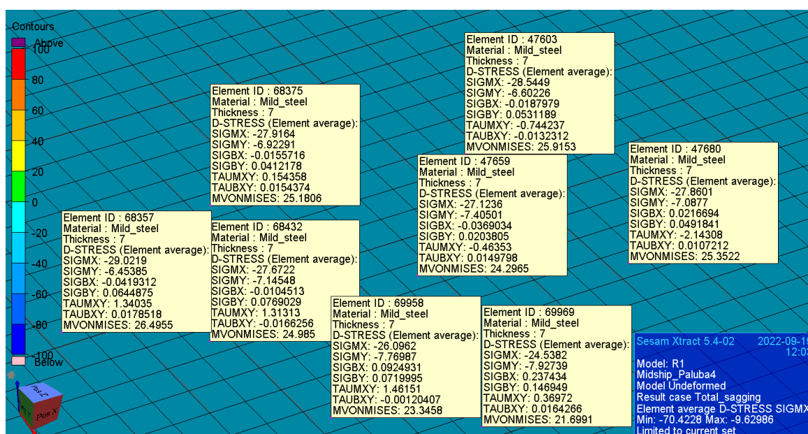
Slika 5.25 Naprezanja Palube 4
