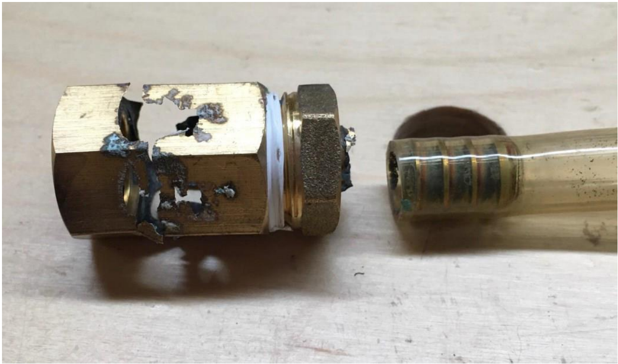
Slika 2.16. Decinkacija mjedi [7]
