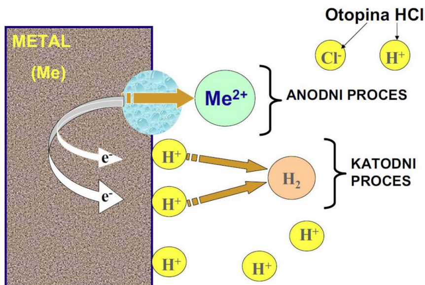
Slika 2.6. Model elektrokemijske korozije [6]
