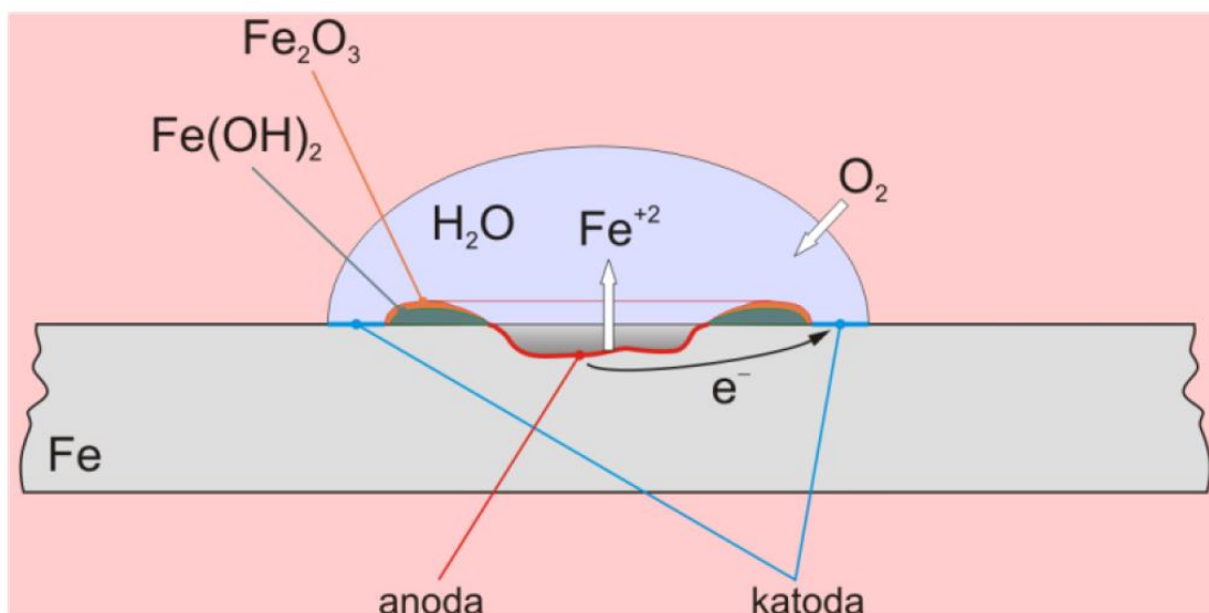
Slika 2.5. Korozija željeza ispod kapi vode [6]
