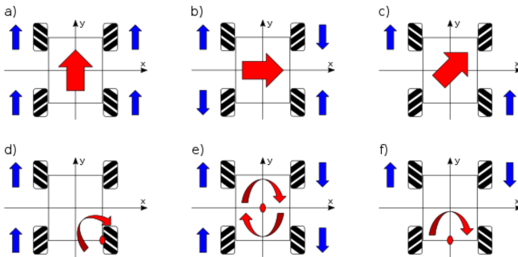
Slika 2.5 Omnidirekcijski pogon sa švedskim kotačima [3]
