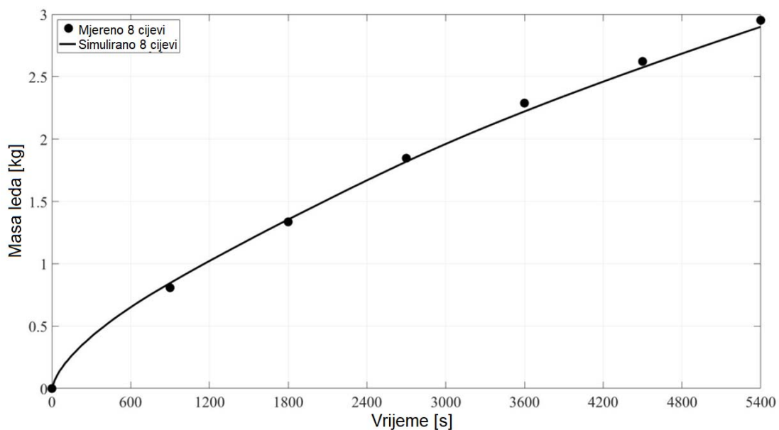
Slika 29. Usporedba mase leda dobivene simulacijom sa masom leda izmjerenom eksperimentom (inicijalna temperatura vode 4^{\circ}\text{C} ) [76]
