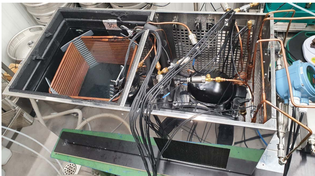
Slika 9. Ispitni uzorak premix rashladnog uređaja
