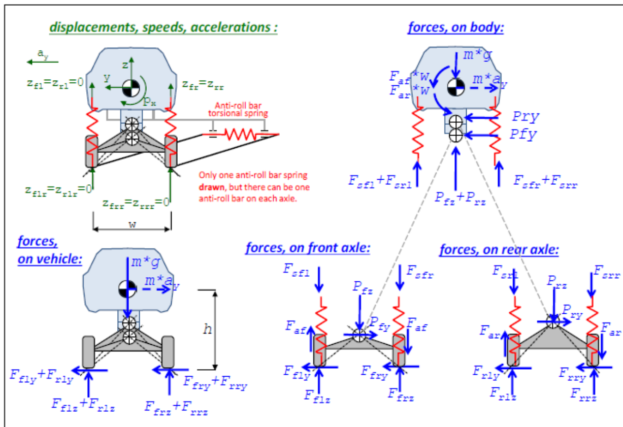
Slika 3.18 Model ravnomjernog uzdizanja i valjanja zbog bočnog ubrzanja, korištenjem središta valjanja, koji mogu biti različiti prednji i stražnji. Uključujući stabilizator na svakoj osovini.
