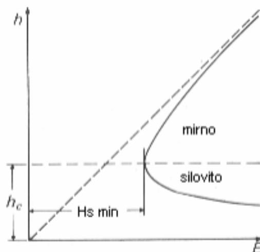
Slika 2.2: Krivulja specifične energije [2]
