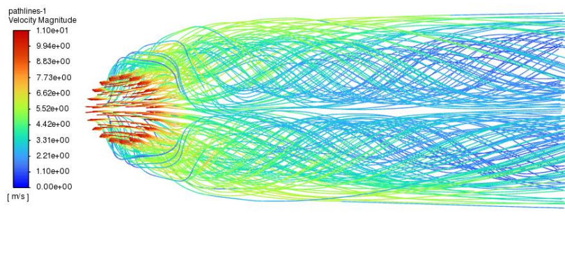
Slika 6.8. Strujnice brzine kod originalnog difuzora
