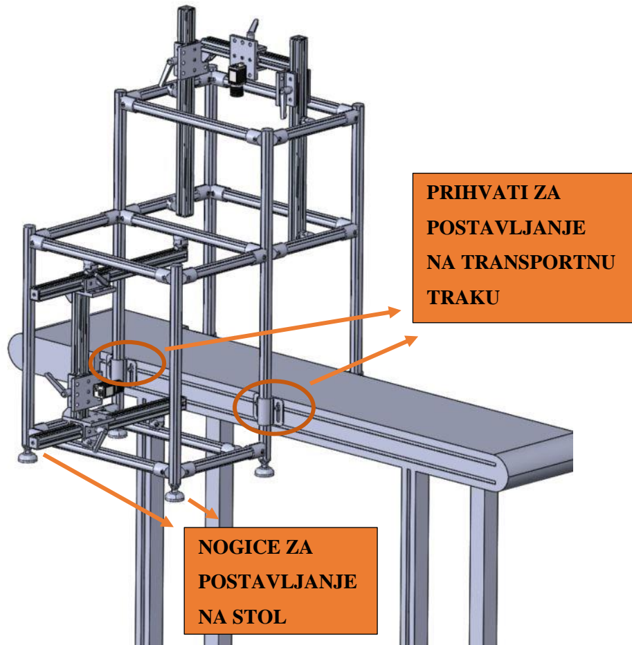
Slika 3.17 Model rekonfigurabilnog sustava
