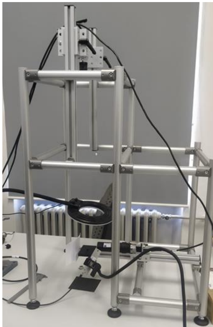
Slika 3.39 Izvedeni RMS postavljen na radnom stolu u laboratoriju
