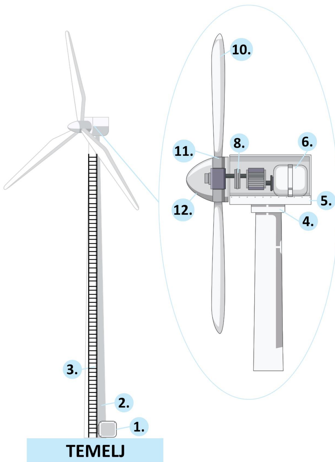
Slika 3.6 Dijelovi vjetroagregata
