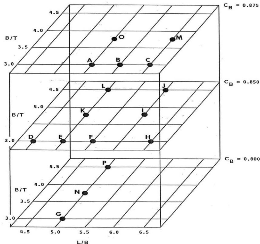
Slika 2.5. Bezdimenzijske serije modela brodskih formi [1]
