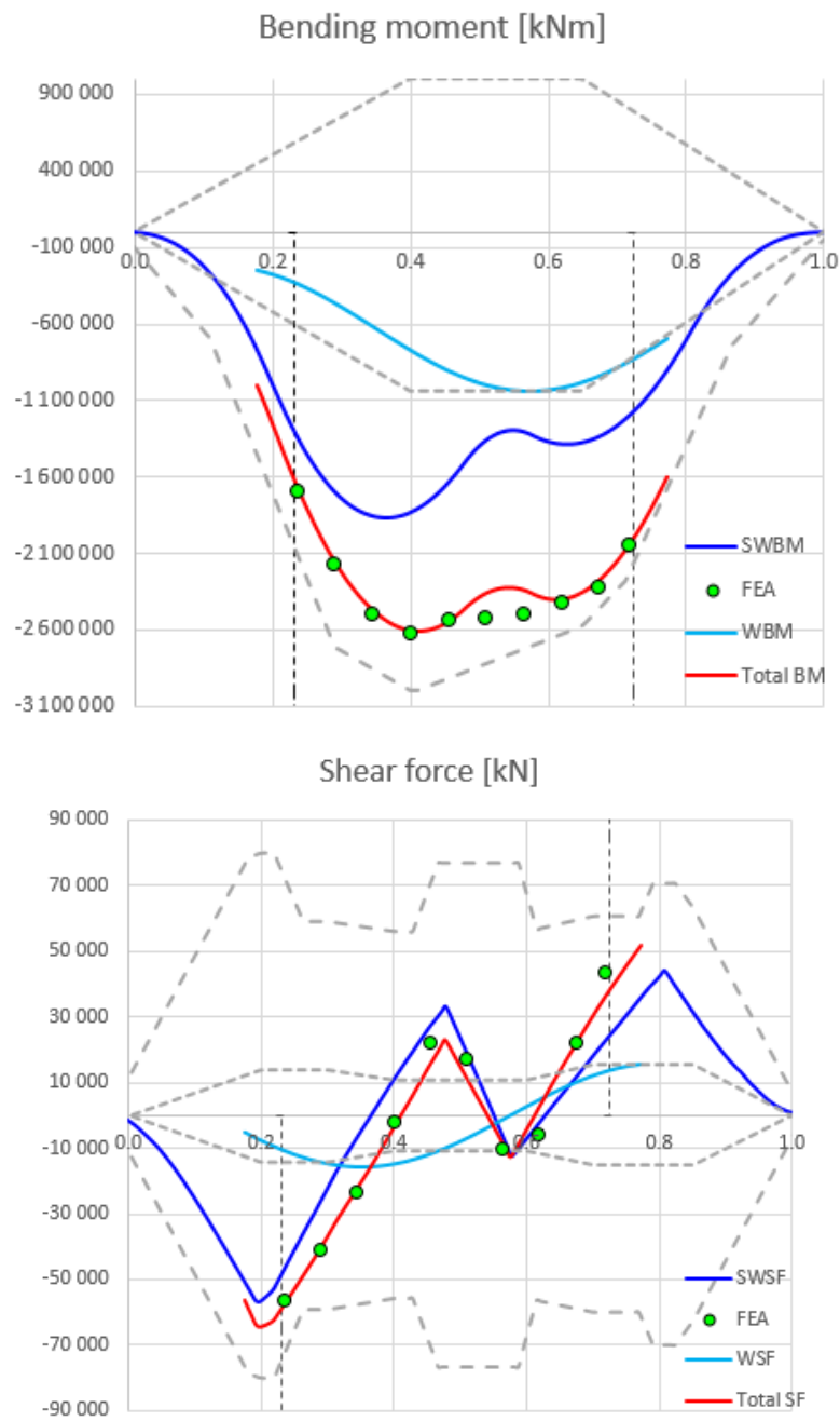
Figure 91 FEA Model loading condition validation – example symmetrical sagging loading Slika 84 FEA model – validacija stanja krcaanja – primjer simetričnog progibnog opterećanja
