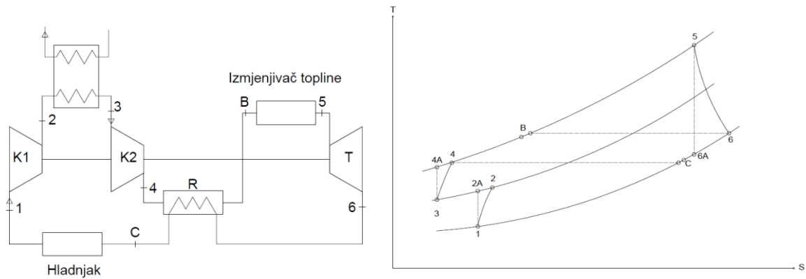
Slika 30. Shema i T-s dijagram zatvorenog sustava plinske turbine u kombinaciji sa međuhlađenjem i regeneratom topline
