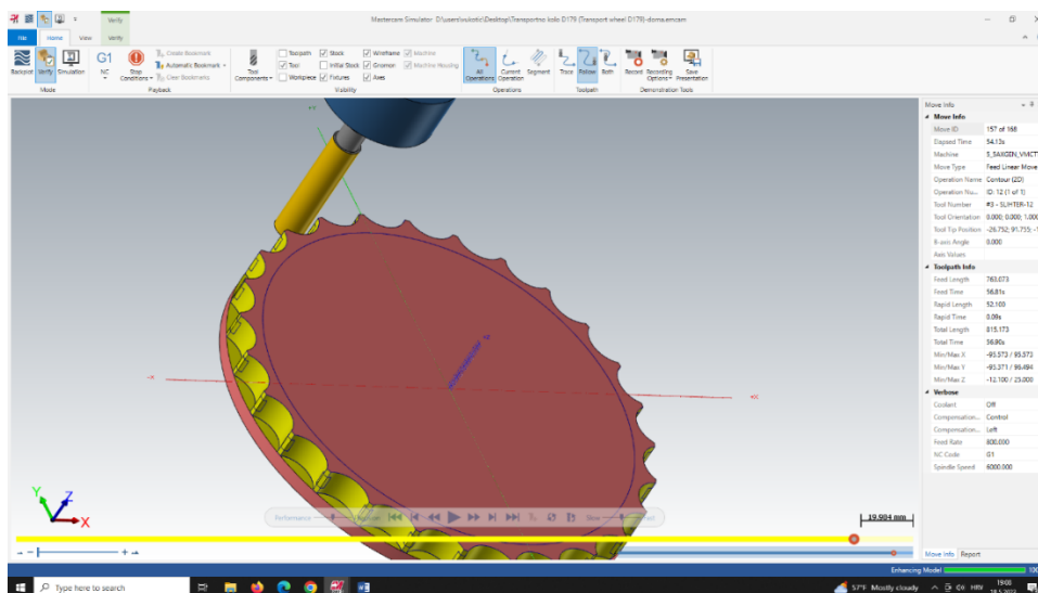
Slika 7.118. Simulacija (OP110)
