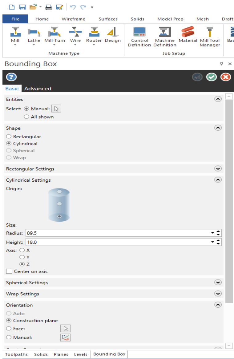
Slika 7.77. Definiranje sirovca
