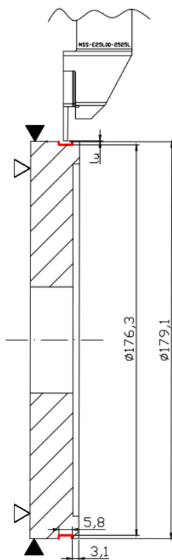
Slika 5.23. Operacija 30 – zahvat 6
