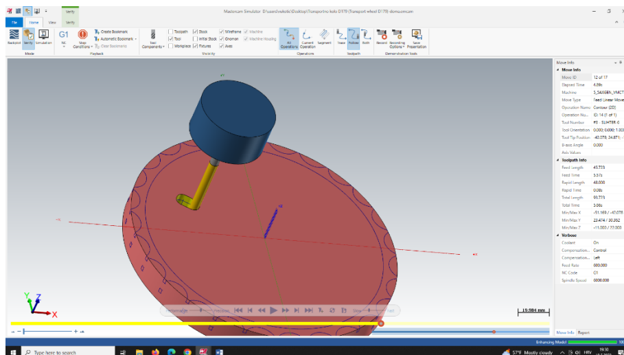
Slika 7.124. Simulacija (OP140)
