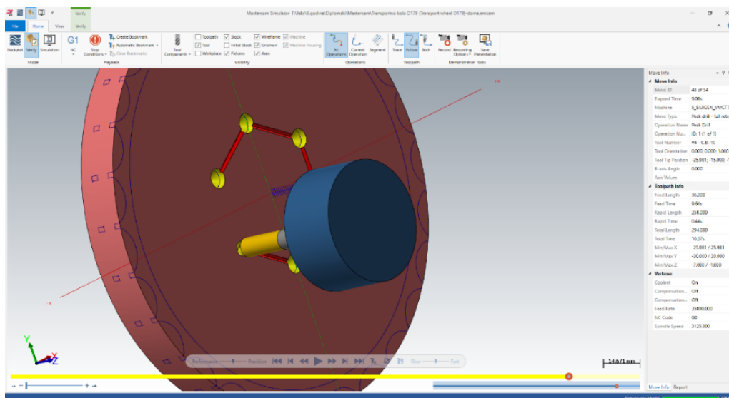
Slika 7.86. Simulacija (OP10)
