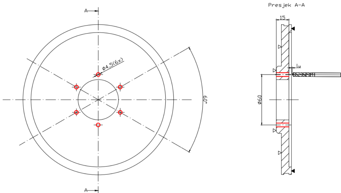
Slika 5.54. Operacija 50 - zahvat 4
