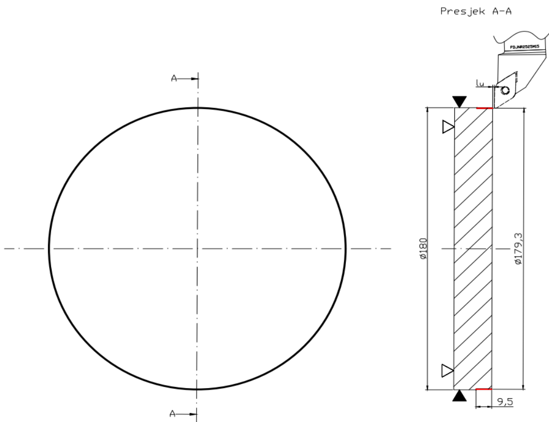
Slika 5.10. Operacija 20 – zahvat 3
