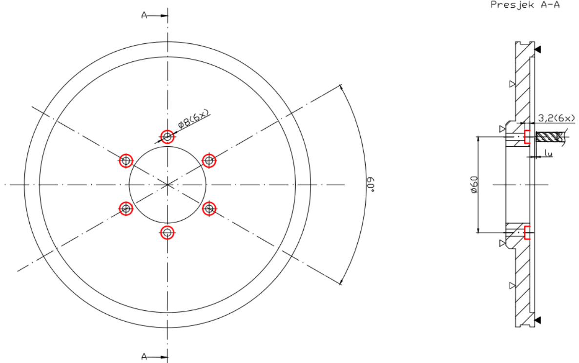
Slika 5.56. Operacija 50 - zahvat 5
