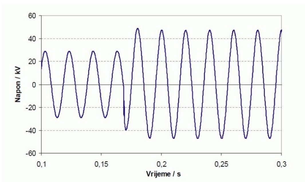
Slika 2.5. Prenapon
