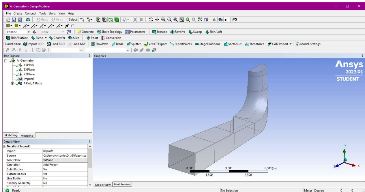
Slika 7.13. Generiranje difuzora
