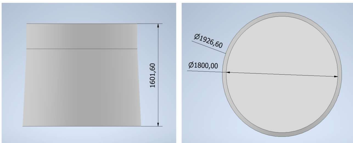
Slika 7.3. Ulaz difuzora
