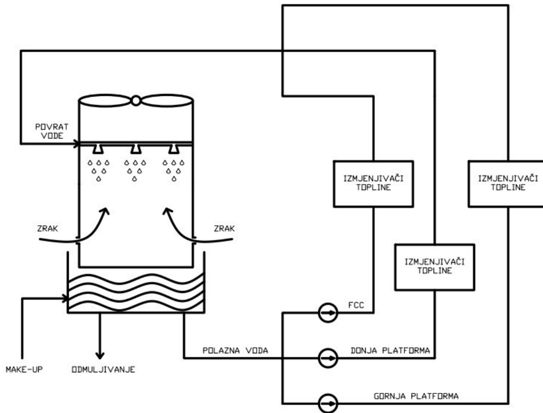
Slika 7.7. Shema postrojenja
