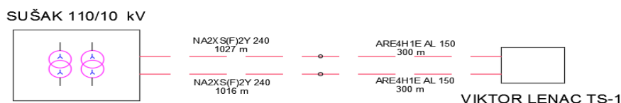
Slika 2.2. Blok shema napajanja Brodogradilišta Viktor Lenac[10]
