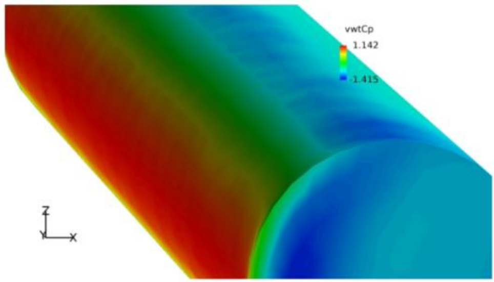
Slika 4.34 : Iznos C_p
