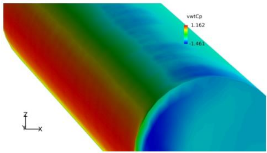
Slika 4.35 : Iznos C_p
