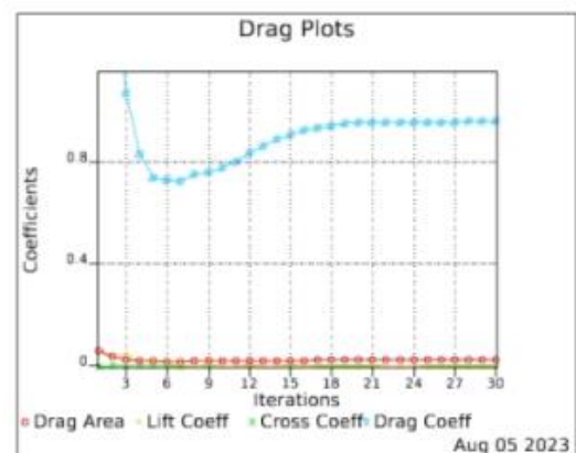
Slika 4.23 : Konvergiranje koeficijenata
