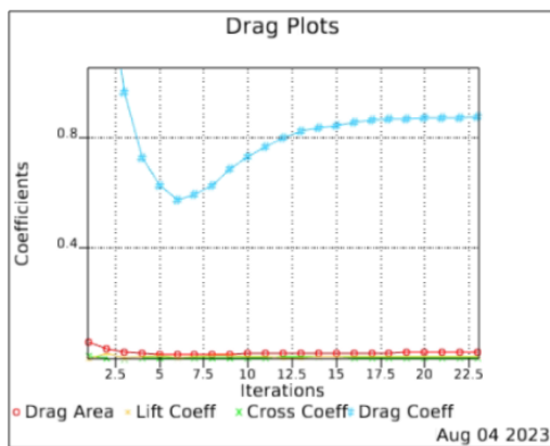
Slika 4.22 : Konvergiranje koeficijenata
