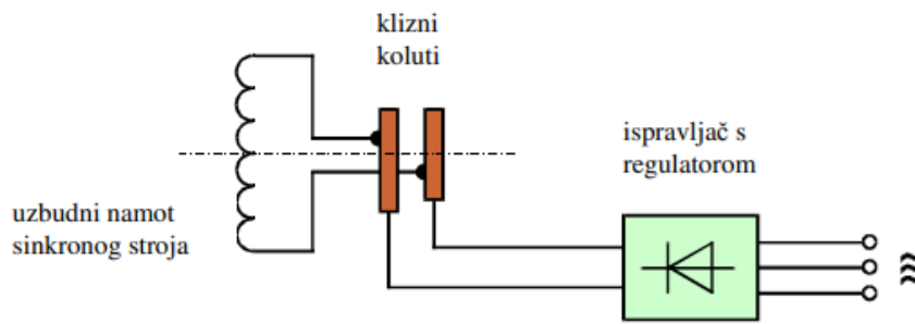
Slika 2.7. Statička uzbuda [2]
