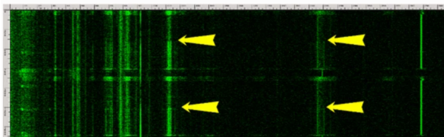
Slika 2.4 Akustični potpis dva GnuPG RSA potpisa (žutim strelicama označeni su prijelazi između p i q ) [1]
