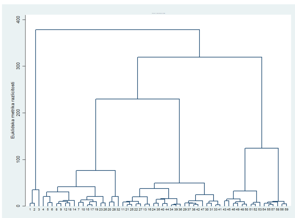
Slika 6.7. Rezultirajući dendrogram
