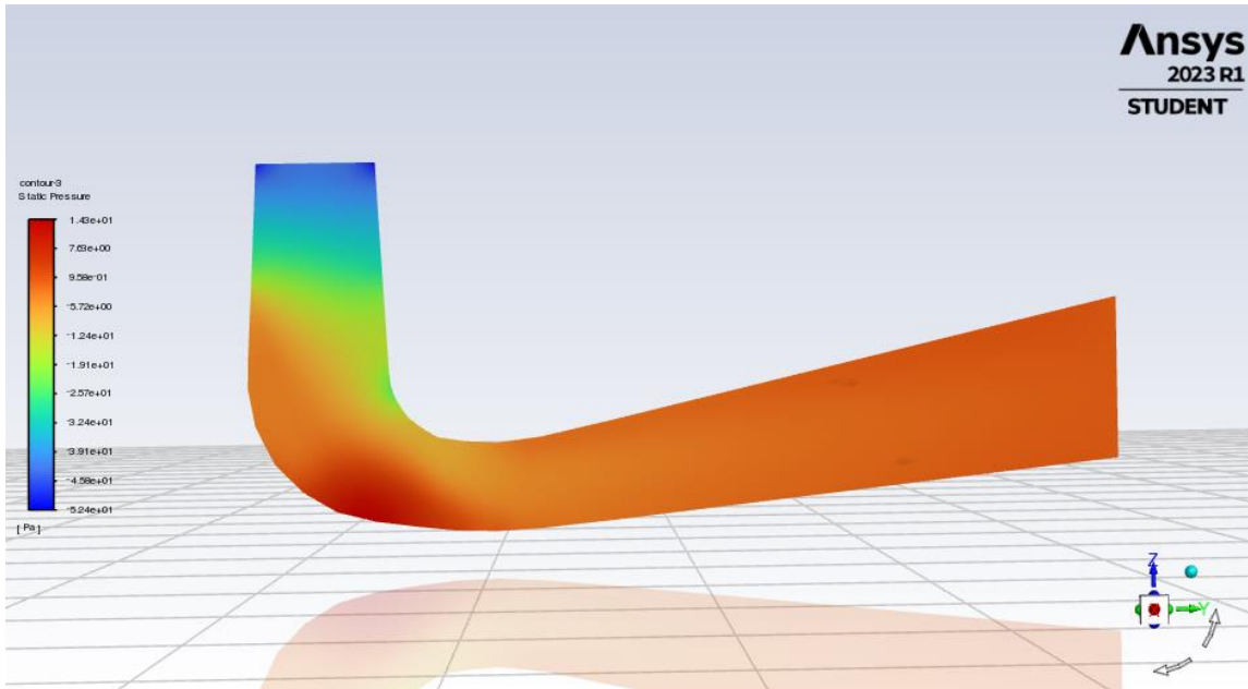
Slika 6.4. Raspodjela statičkog tlaka po presječnoj YZ ravnini difuzora
