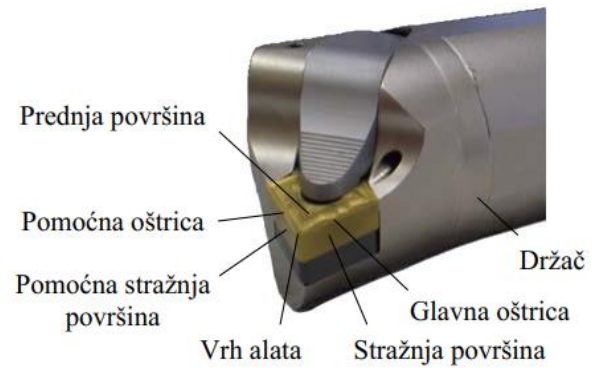
Slika 2.1.2. Rezni klin alata, površine i oštrice alata [1].
