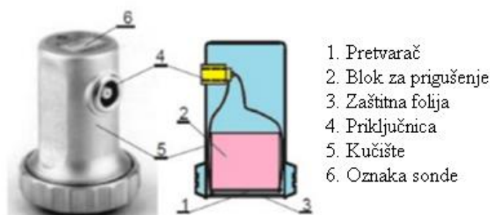
Slika 6.8. Ravna sonda [19]
