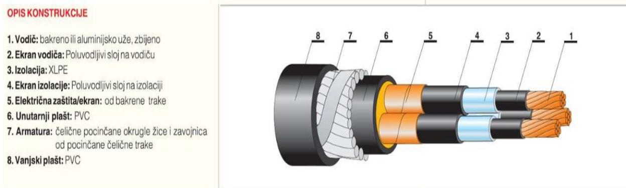
Slika 2.24. Prikaz trožilnog srednjonaponskog elektroenergetskog kabela s XLPE izolacijom i PVC plaštom s pripadajućim opisom konstrukcije [20]
