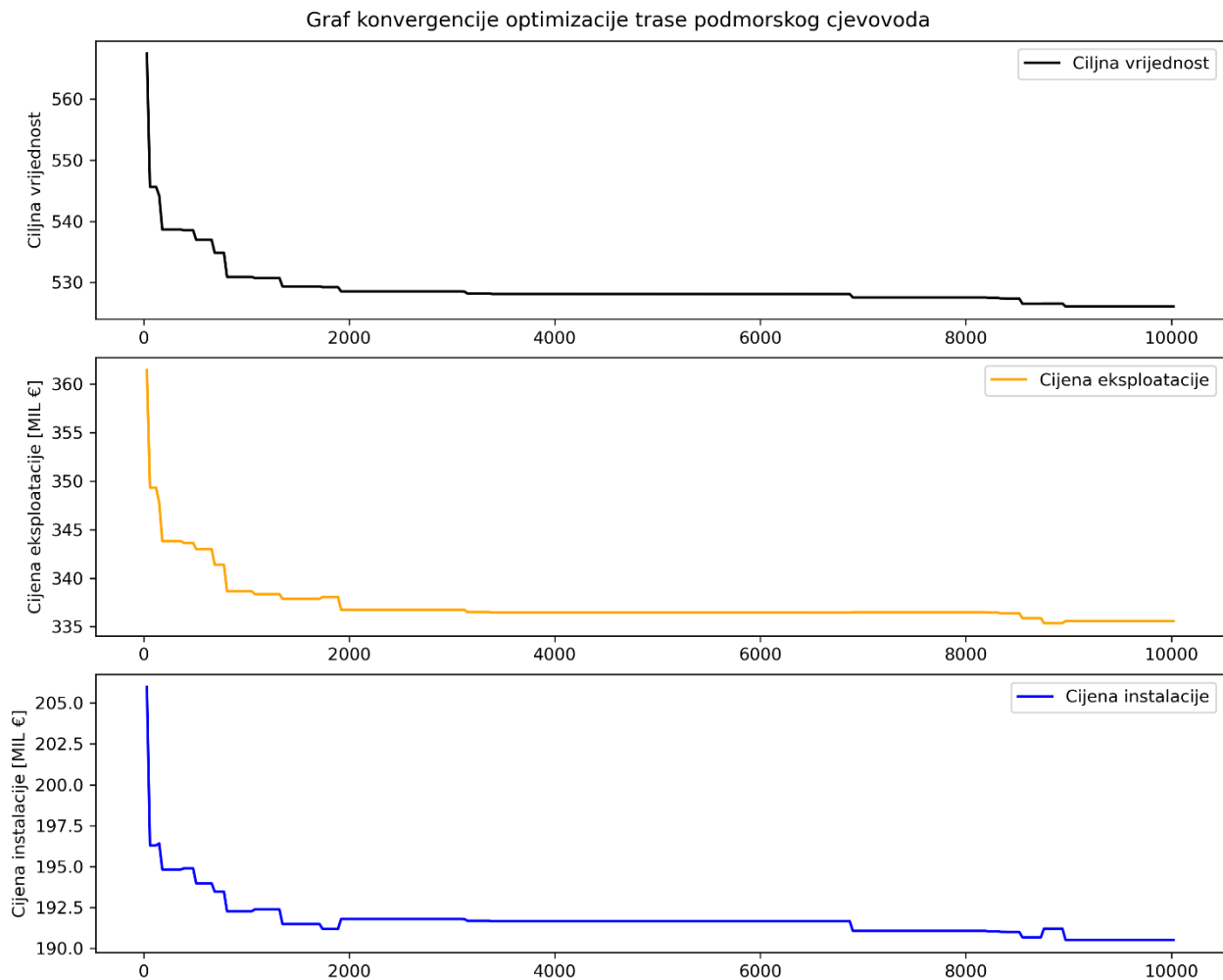
Slika 6-1. Graf konvergencije pri optimizaciji trase podmorskog cjevovoda
