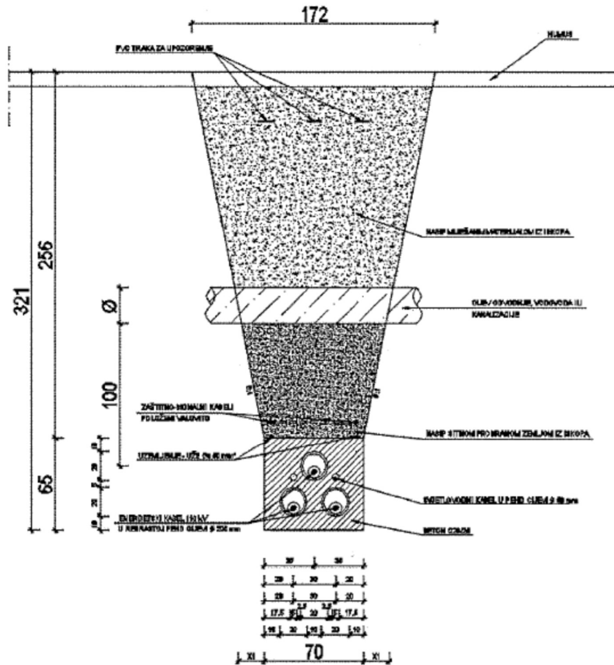
Slika 9.3: Poprečni presjek kabelskog rova s podzemnim kabelima smještenim u zaštitnim PEHD cijevima promjera 200 mm u zaštitnom betonskom bloku na točki najdublje smještenih kabela na križanju s evidentiranom instalacijom kanalizacije [7]
