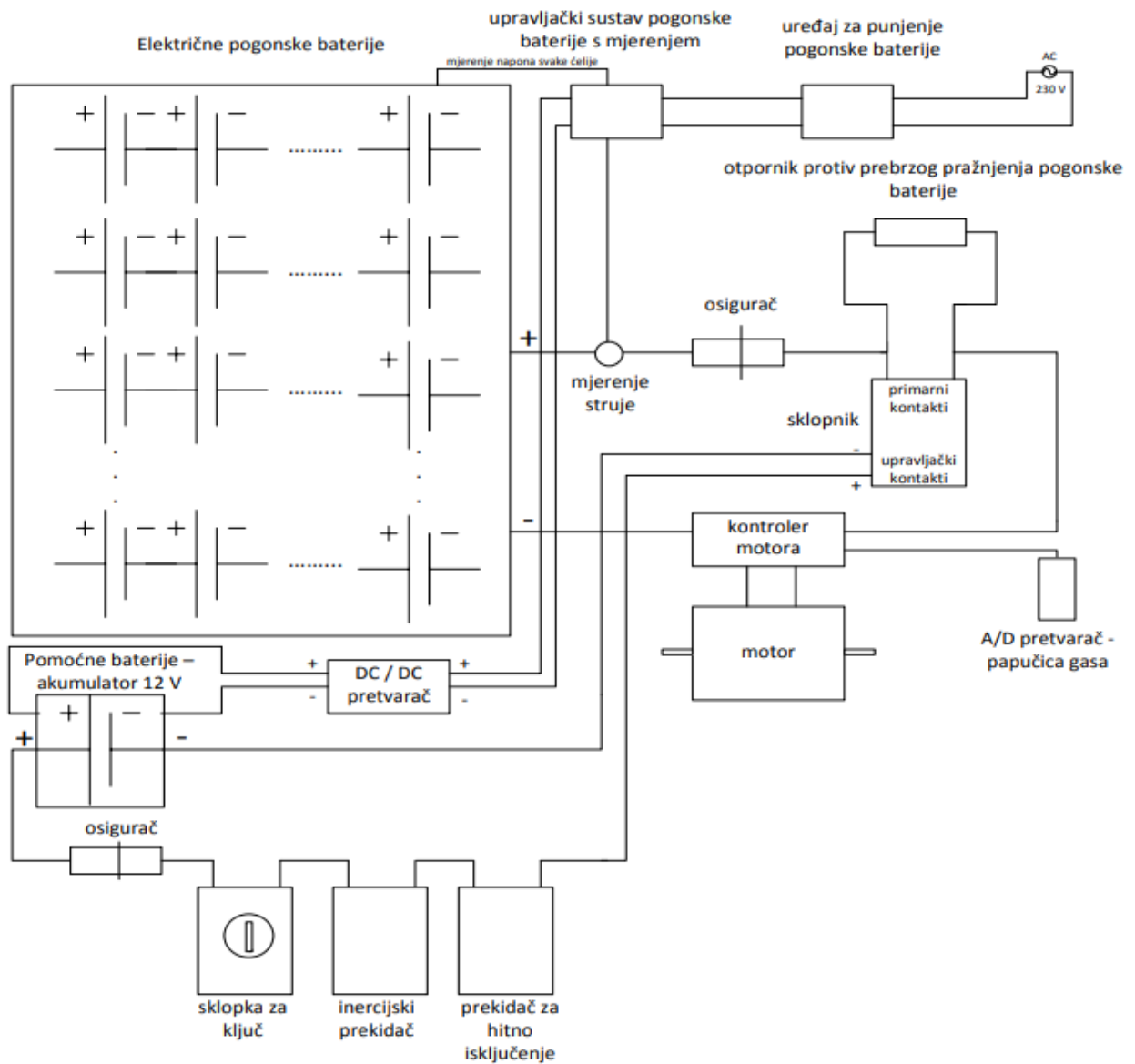
Slika 2.7. Blok shema elemenata vozila na električni pogon
