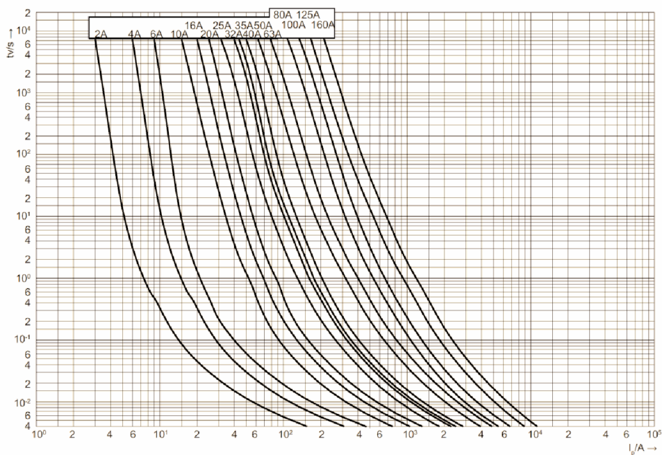
Slika 5.7 Vremensko strujna karakteristika NV osigurač gG, vel. NH000, Schrack [8]
