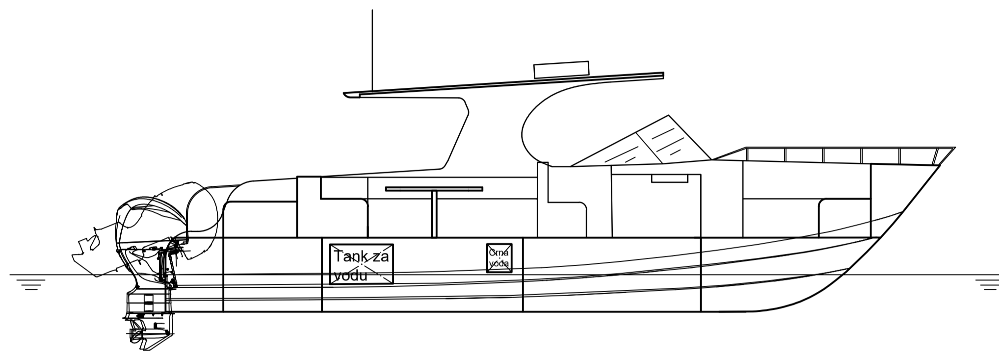
IZVEDBA 2. - S VANBRODOKIM PROPULZORIMA - POGLED NA DESNU STRANU
