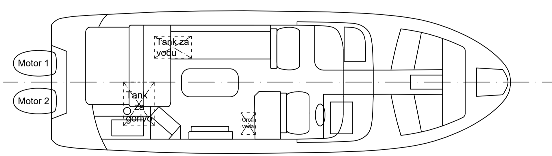
IZVEDBA 2. - S VANBRODOKIM PROPULZORIMA - TLOCRT GLAVNE PALUBE
