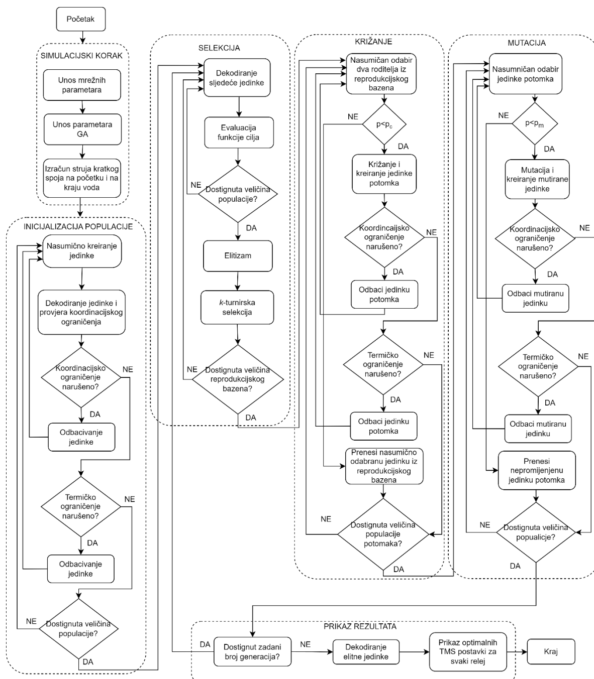
Slika 7.13 Dijagram razvijenog optimizacijskog algoritma
