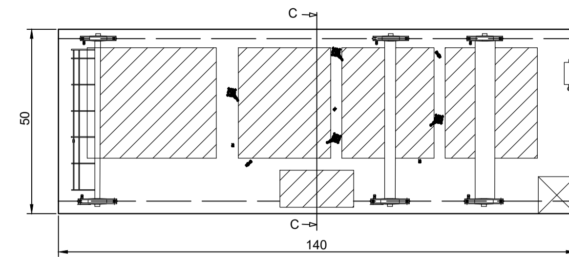
Radionica predmontaže
