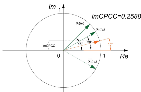
Slika 5.6: Vizualizacija izračuna imCPCC za pojedini uzorak.
