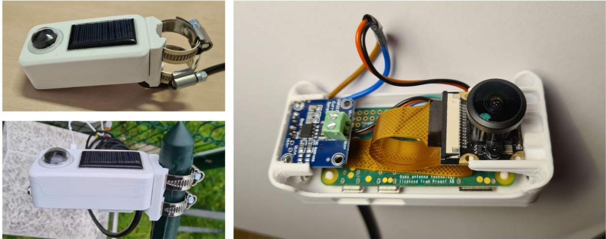
Slika 11: Sastavljeni modul
