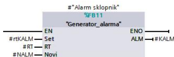
Slika 2.5 Izgled funkcijskog bloka generatora alarma
